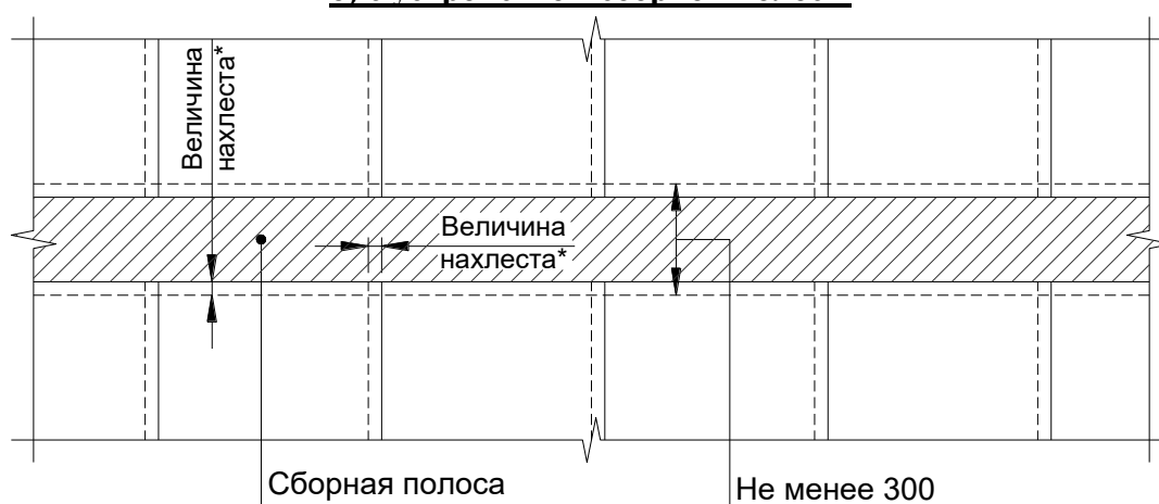
Рисунок 6.1 – Варианты раскладки полотен битумосодержащих материалов
