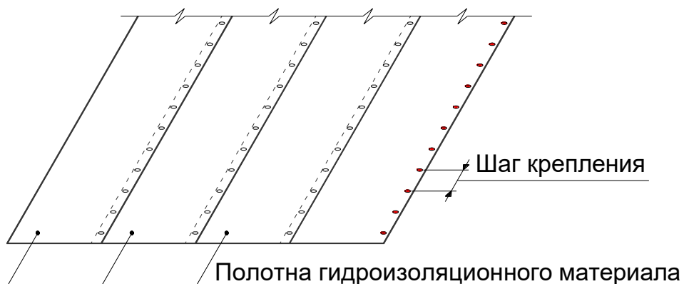
Рисунок 6.5 – Стандартная схема установки крепежа
