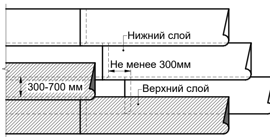
Рисунок 6.4 – Смещение полотен рулонных битумосодержащих материалов в смежных слоях
