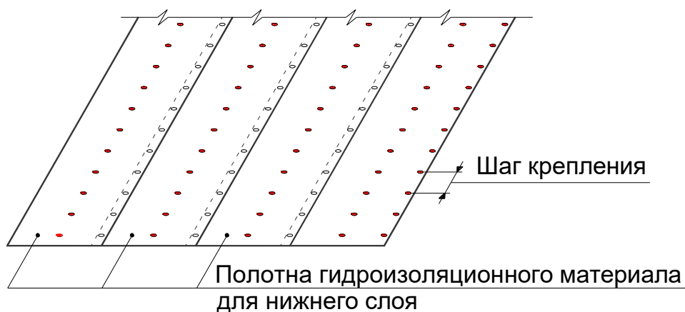
Рисунок 6.6 – Схема крепления материалов по центру рулона
